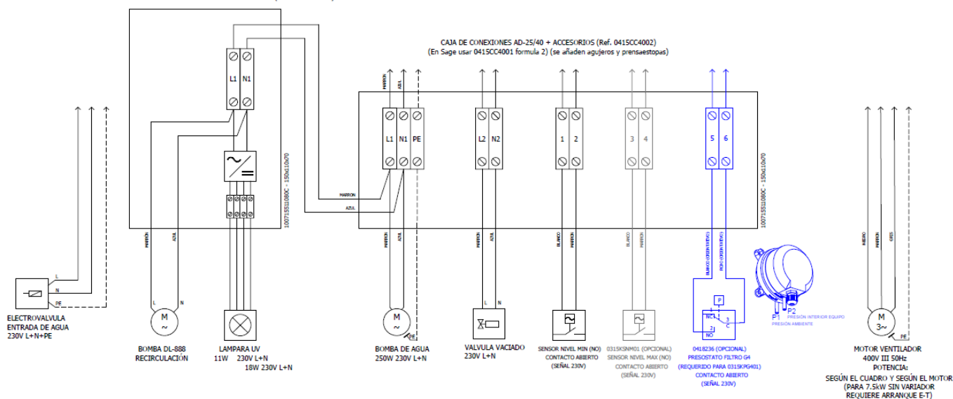
CAJA DE CONEXIONES LAMPARA UV & BOMBA RECIRCULACIÓN (Ref. 0415CUUV01)
