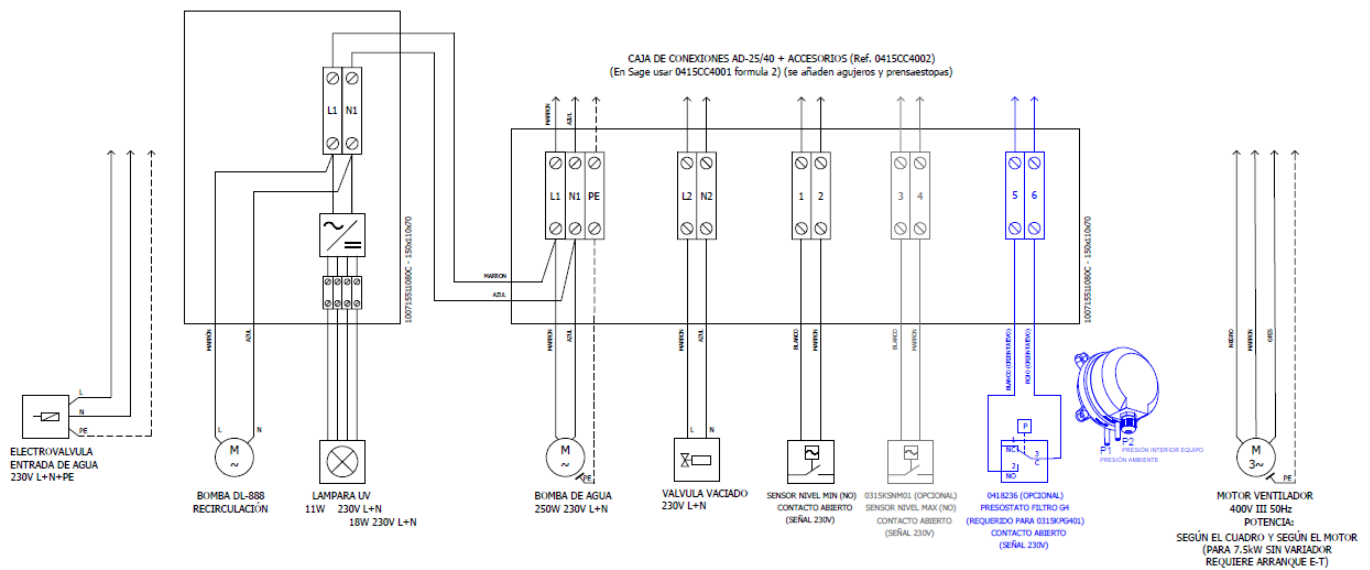
CAJA DE CONEXIONES LAMPARA UV & BOMBA RECIRCULACI  N (Ref. 0415CCUV01)
