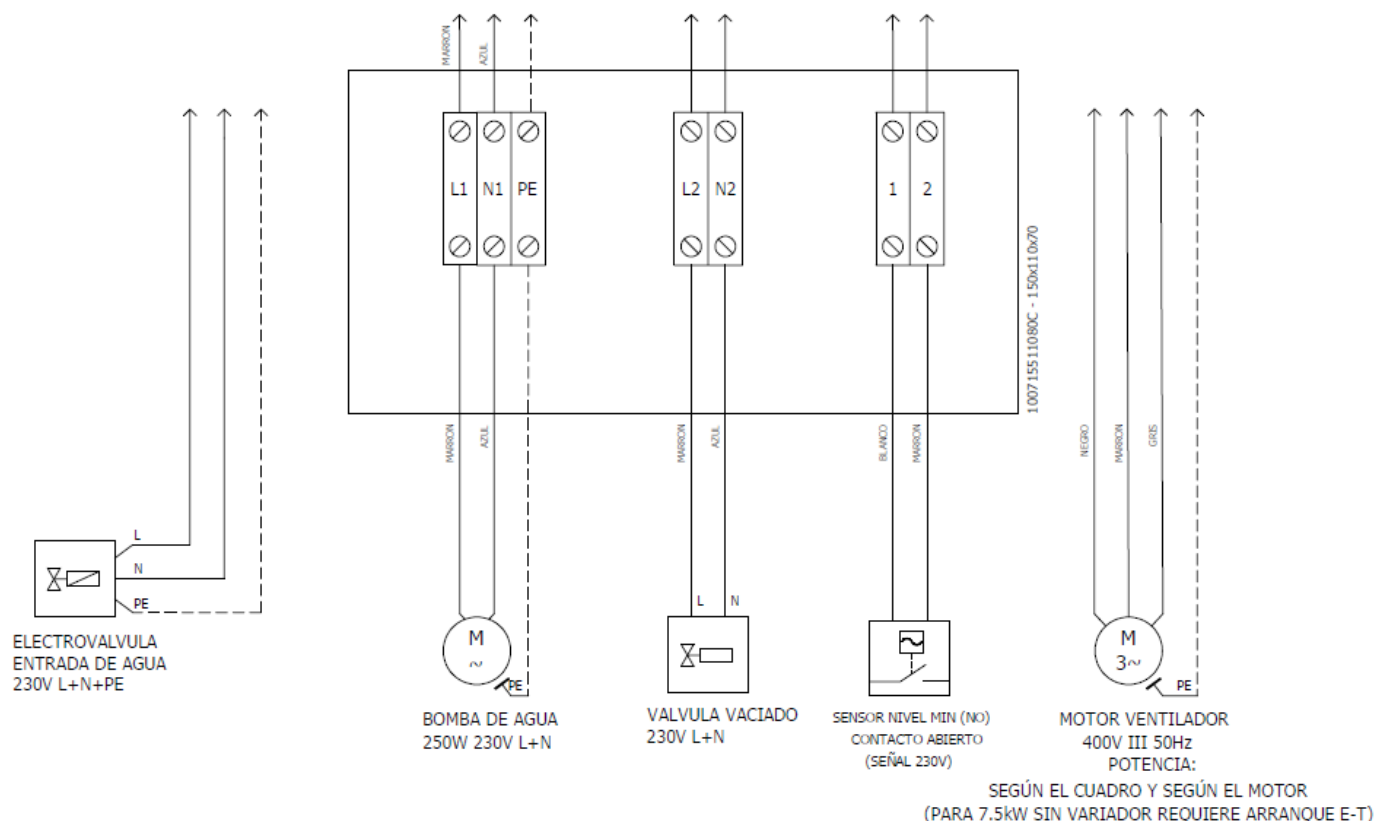
CAJA DE CONEXIONES AD-25/40 (Ref. 0415CC4001 - 0421567)
