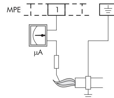
Μικροαμπερομετρική σύνδεση
