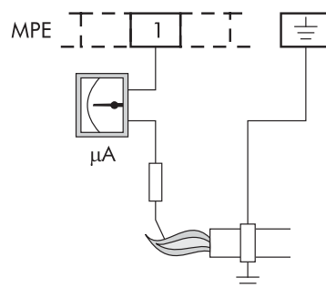
CONEXIÓN MICROAMPERÍMETRO
