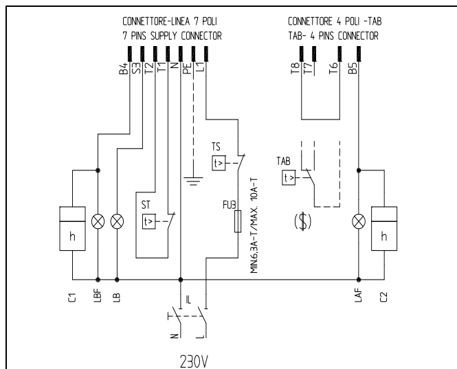
Fig. 27 - Conectores 7 y 4 polos
