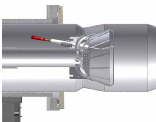
Fig. 36 - Posici3n "toda hacia adelante"
