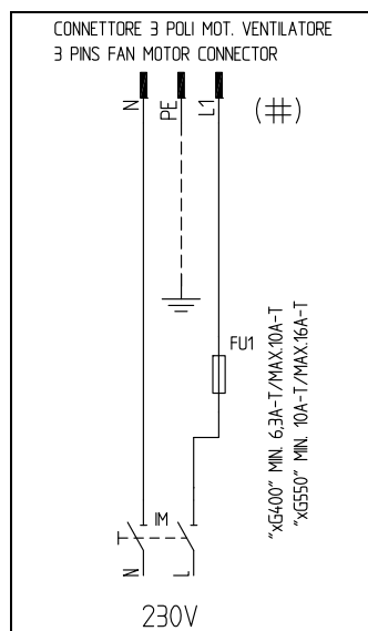
Fig. 26 - Conector 3-polos por el motor eléctrico
