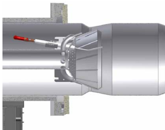
Fig. 37 - Posici3n "toda hacia atràs"
