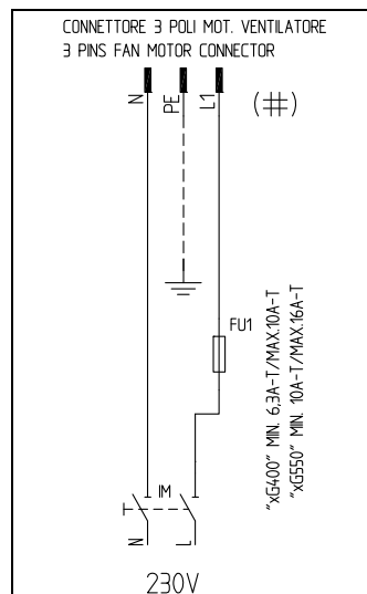
Fig. 28 - Conector 3-polos por motor eléctrico
